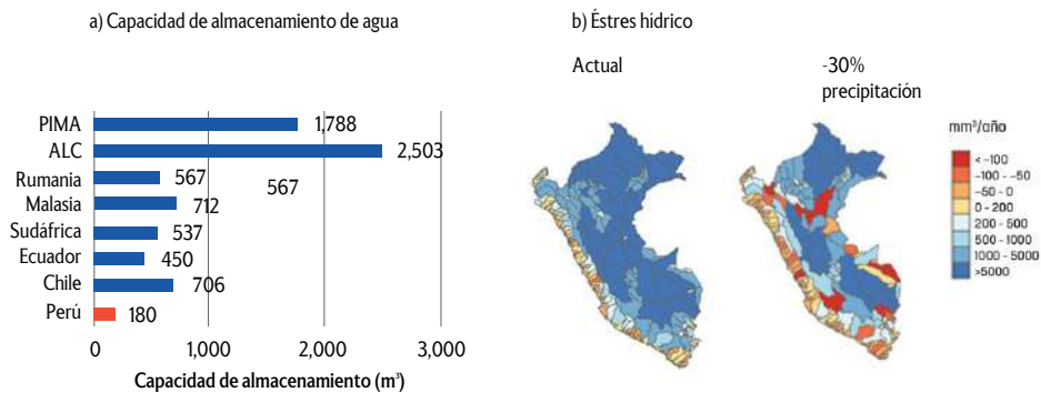
Gráfico 3.24 Capacidad de almacenamiento de agua y estrés hídrico en Perú
