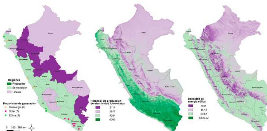
Gráfico 3.19 Ubicación y potencial de las fuentes de bioenergía, energía solar y energía eólica
